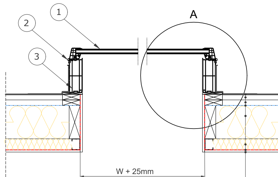
Section A-A' 1:10
