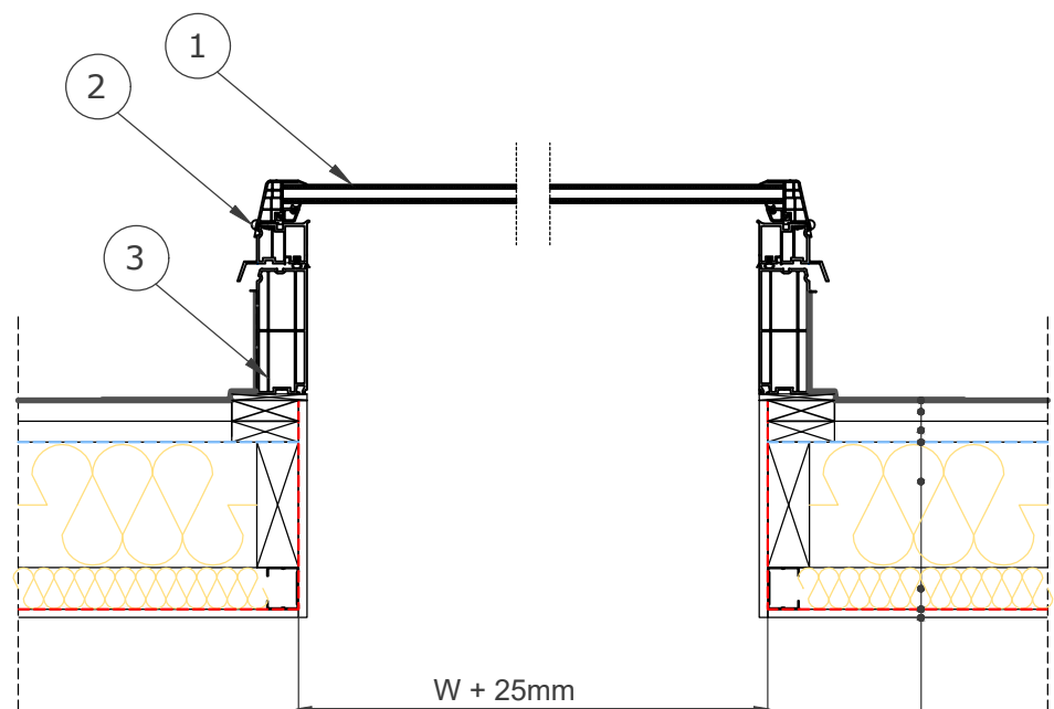
Section A-A' 1:10
