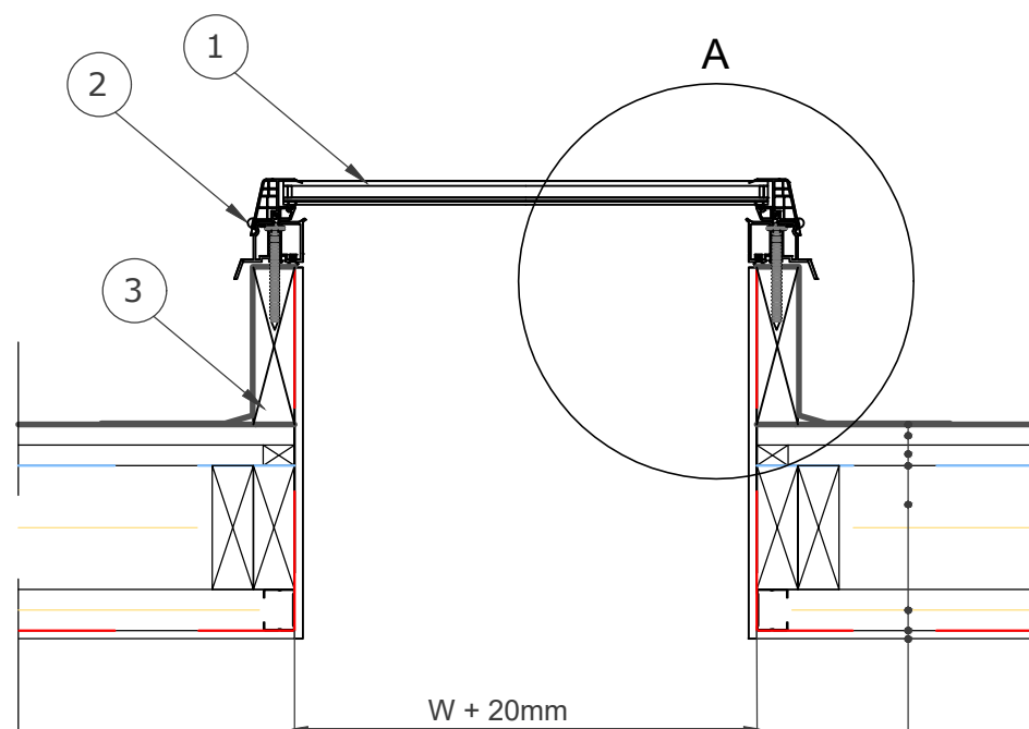
Section A-A' 1:10
