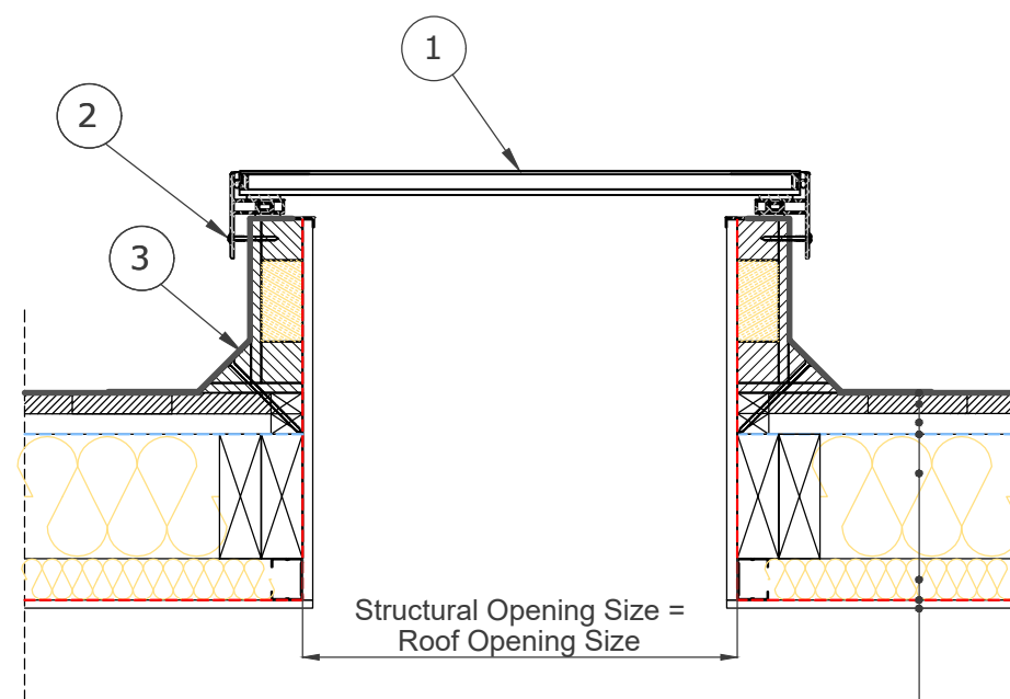
Section A-A' 1:10
