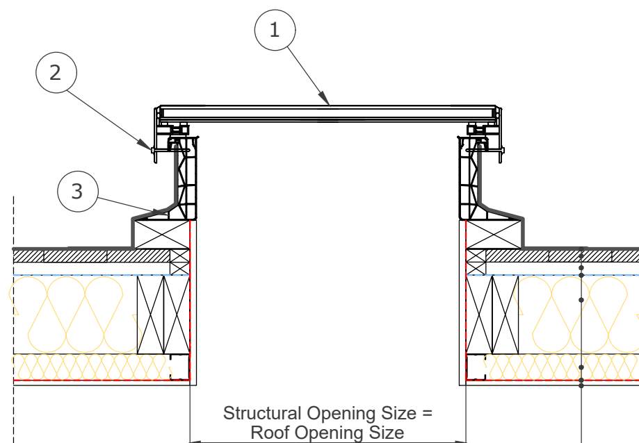
Section A-A' 1:10
