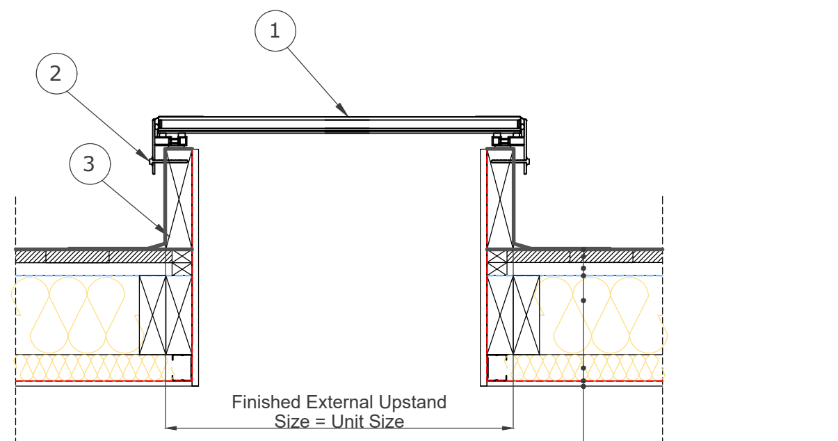
Section A-A' 1:10
