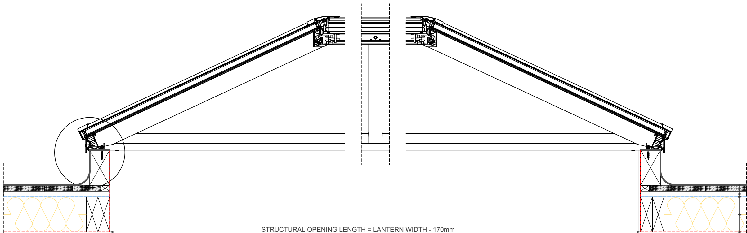
Section A-A' 1:10
