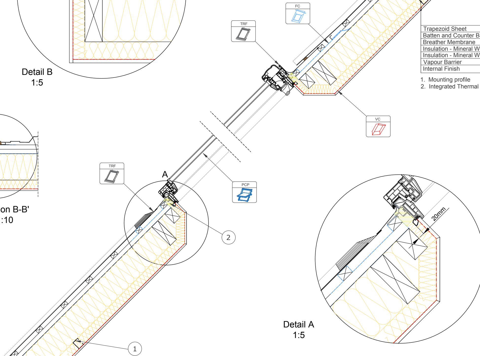
Section A-A' 1:10
