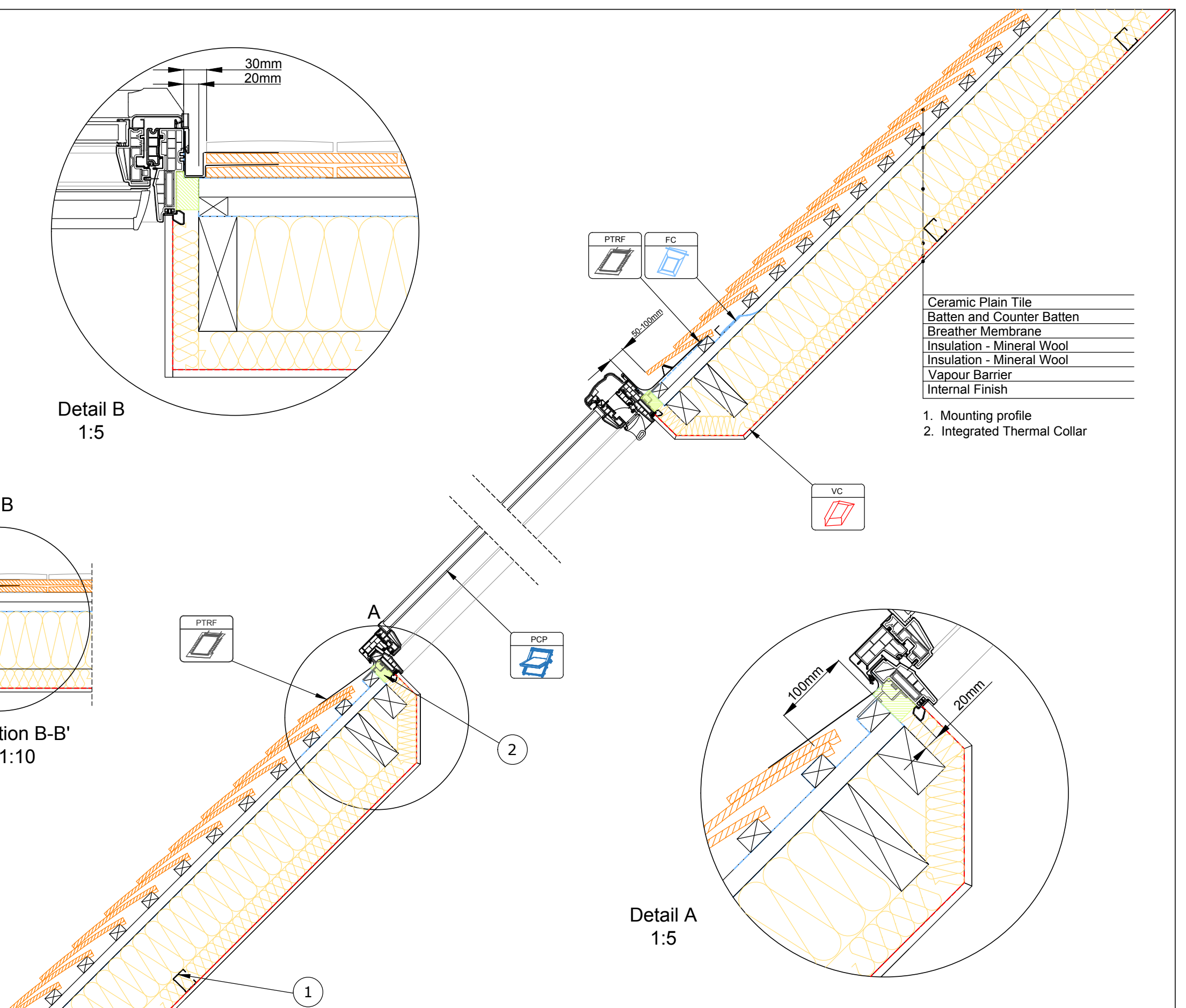
Section A-A' 1:10
