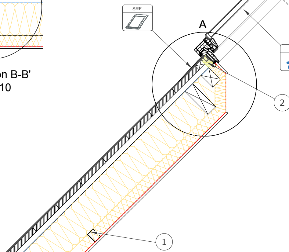
Section A-A' 1:10
