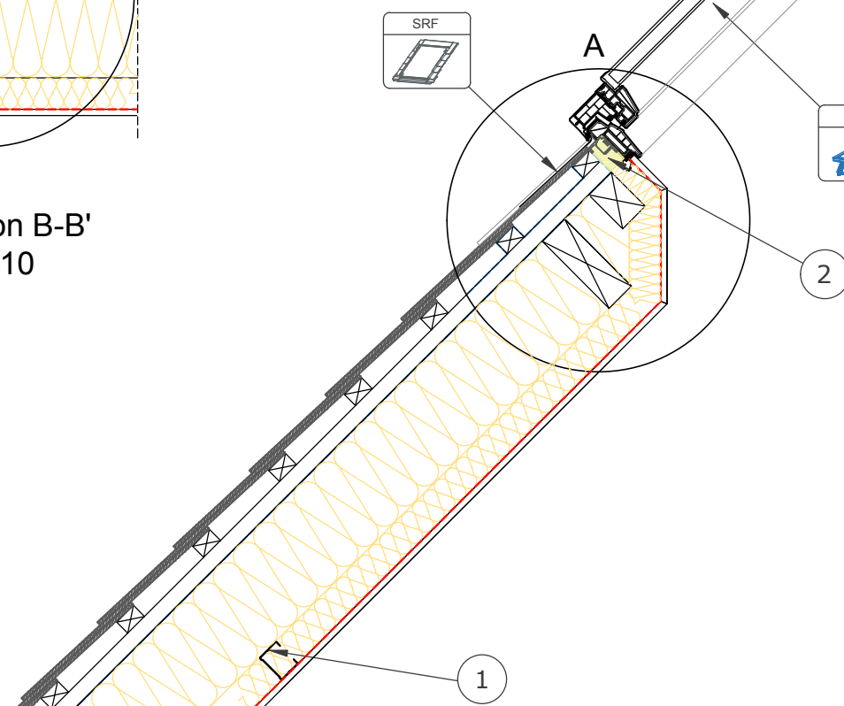
Section A-A' 1:10
