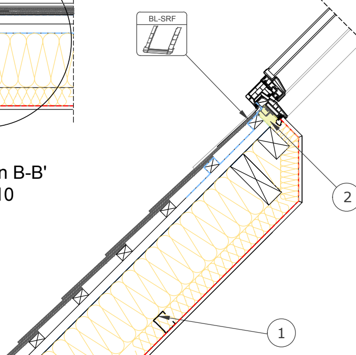
Section A-A' 1:10
