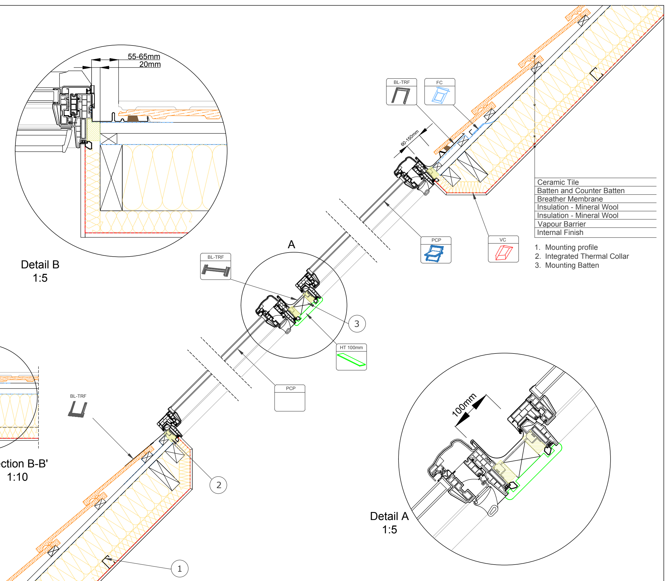
Section A-A' 1:10
