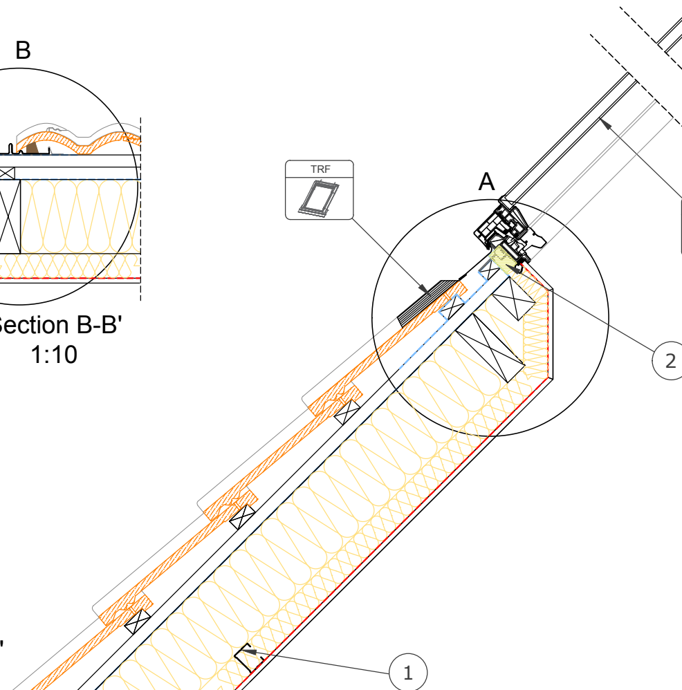
Section A-A' 1:10
