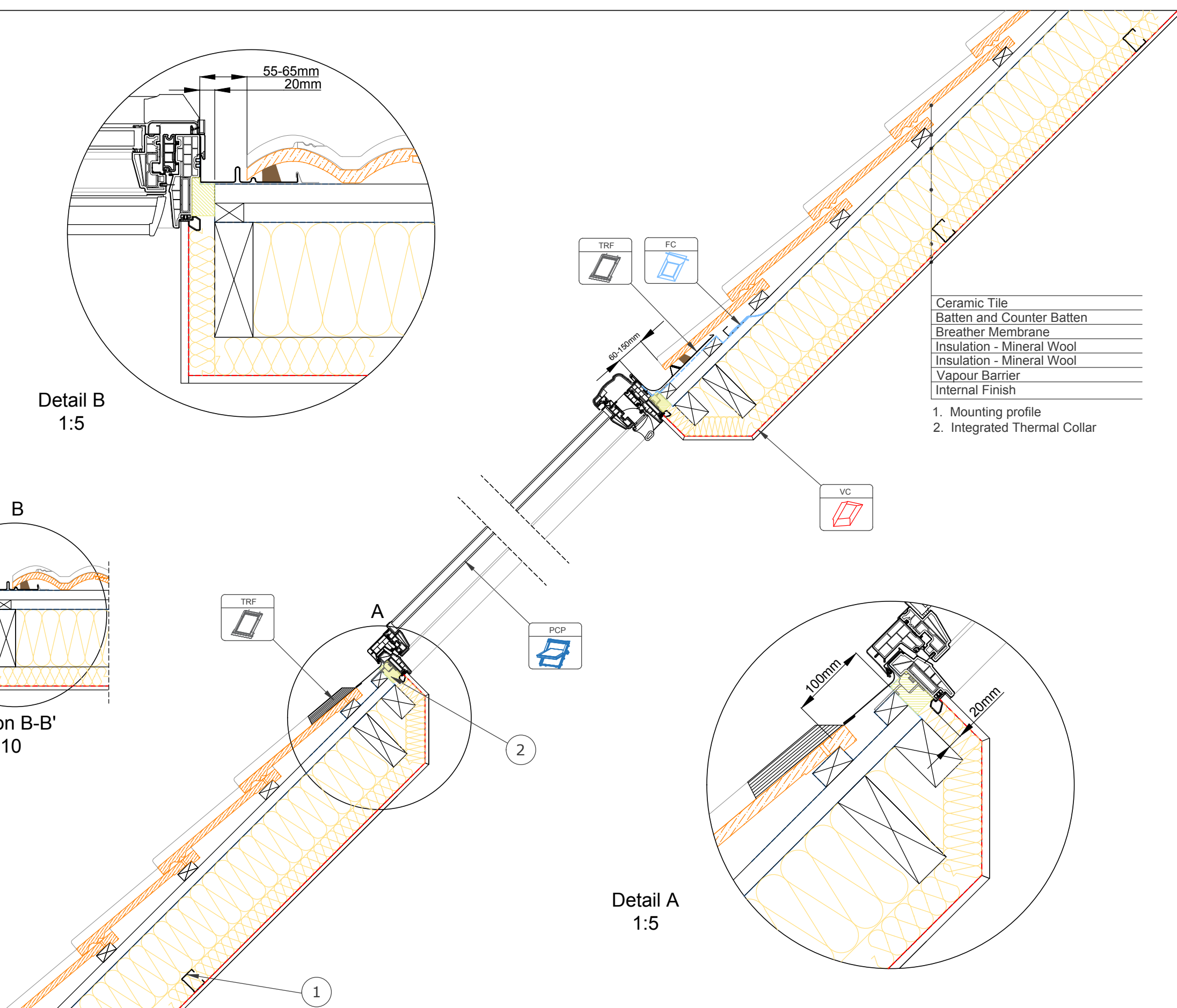
Section A-A' 1:10
